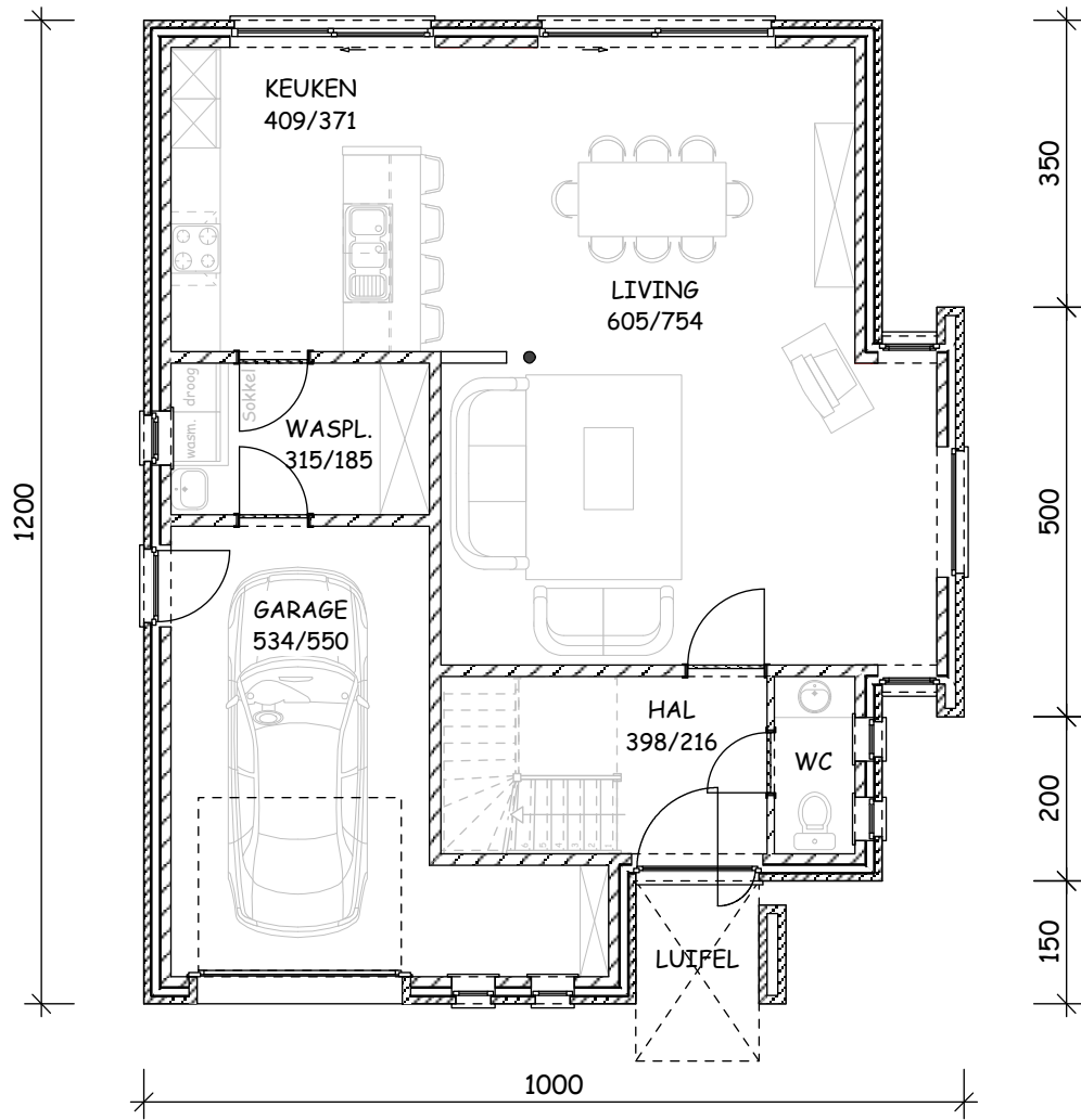
GRONDPLAN
