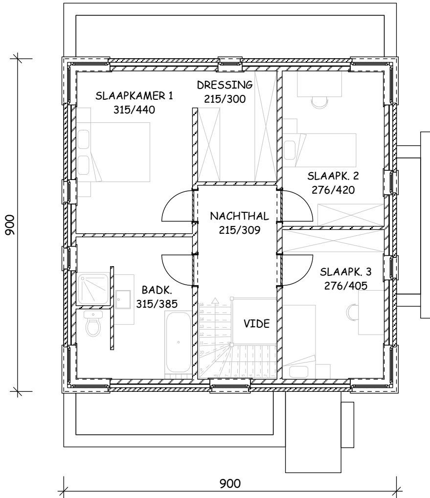
VERDIEPINGSPLAN
